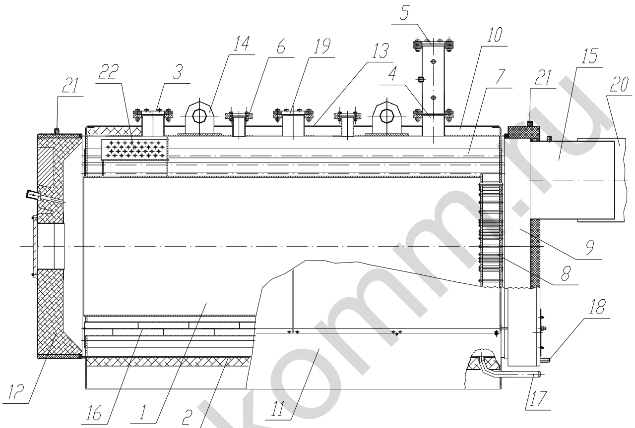
Рисунок 1. Продольный разрез водогрейного котла серии "ЗИОСАБ М"
